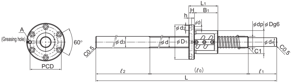
Model BNF
