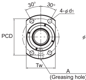
WHF2040,2550/WTF
